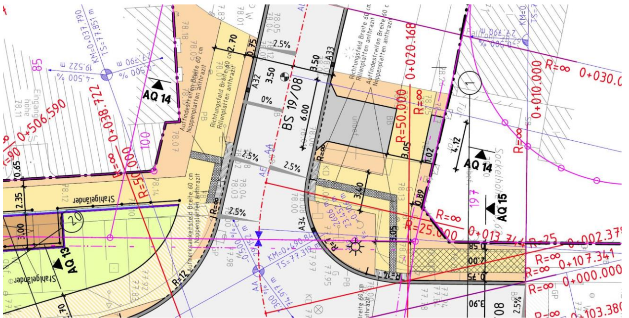
Bild: aus der Planung von 2014 - Querung Breithaus/Drebkauer Straße
